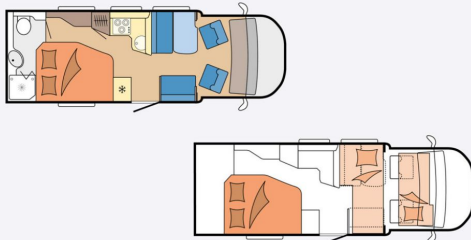
Grundriss Tag/Nacht: Hobby OPTIMA DE LUXE T70 F 2024
